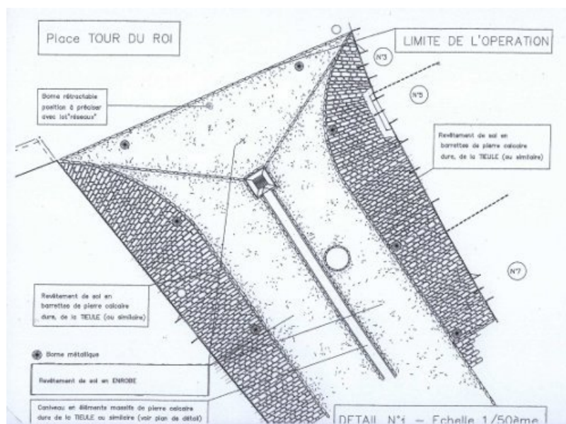
Plan d'aménagement de la rue de la trompe, à l'intersection de la place tour du roi, enrobé et pierre naturelle de Tieule ou similaire s'harmonisent. Dessin C. Espérandieu, architecte.
